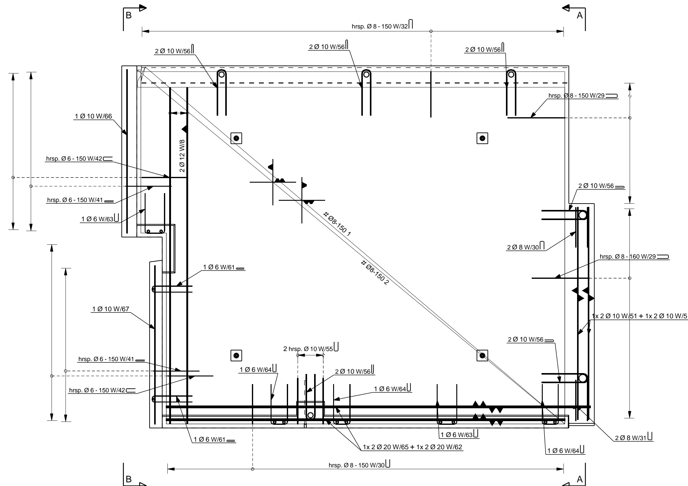
Bovenaanzicht
